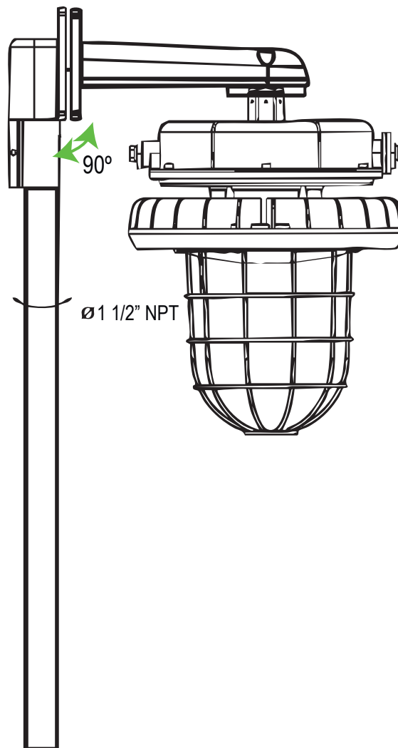
PUNTA DE POSTE 90° CON BRAZO
