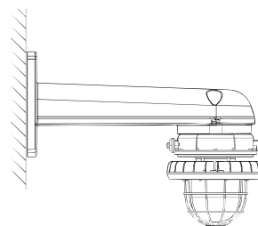
BRAZO con REFRACTOR y con GUARDA.
